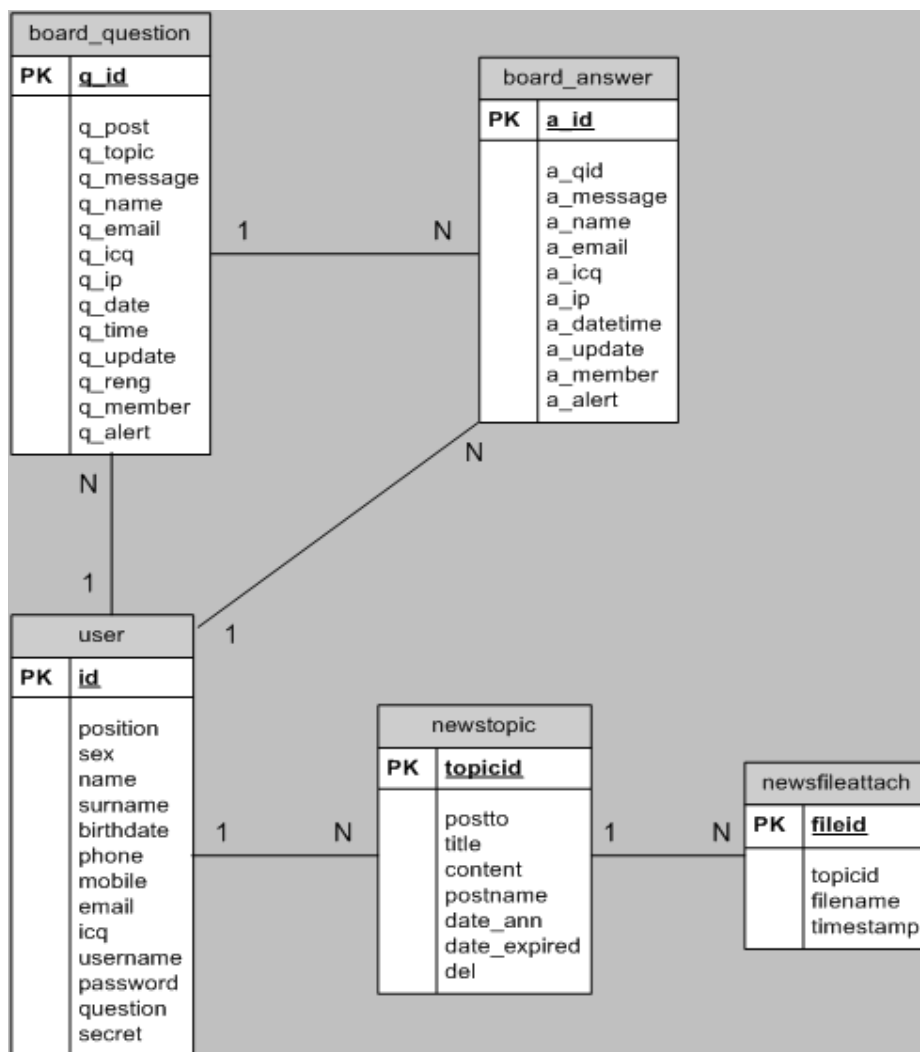
รูปภาพที่ 3.31 แสดงความสัมพันธ์ของตารางทั้งหมดในฐานข้อมูล
