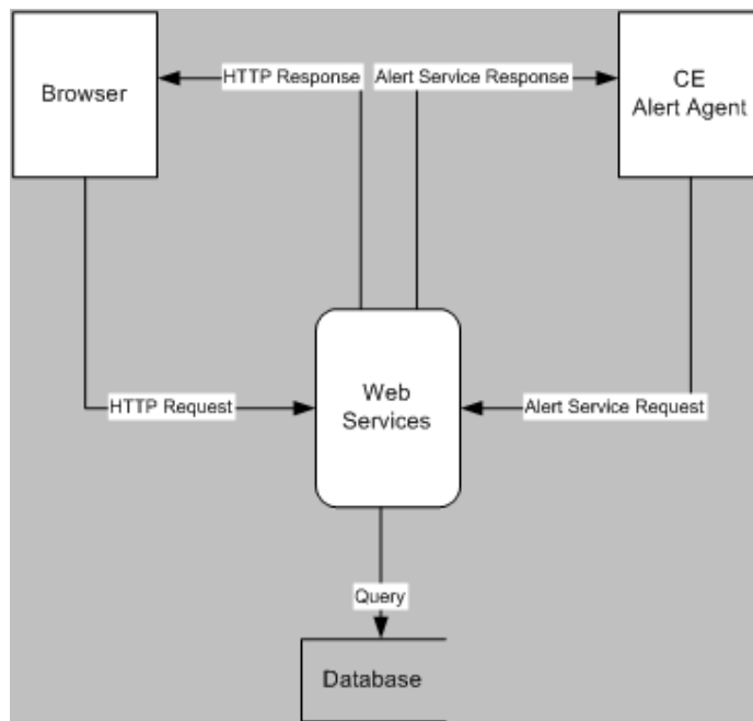
รูปภาพที่ 3.1 Context Diagram
